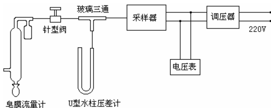
图 1连接示意图
