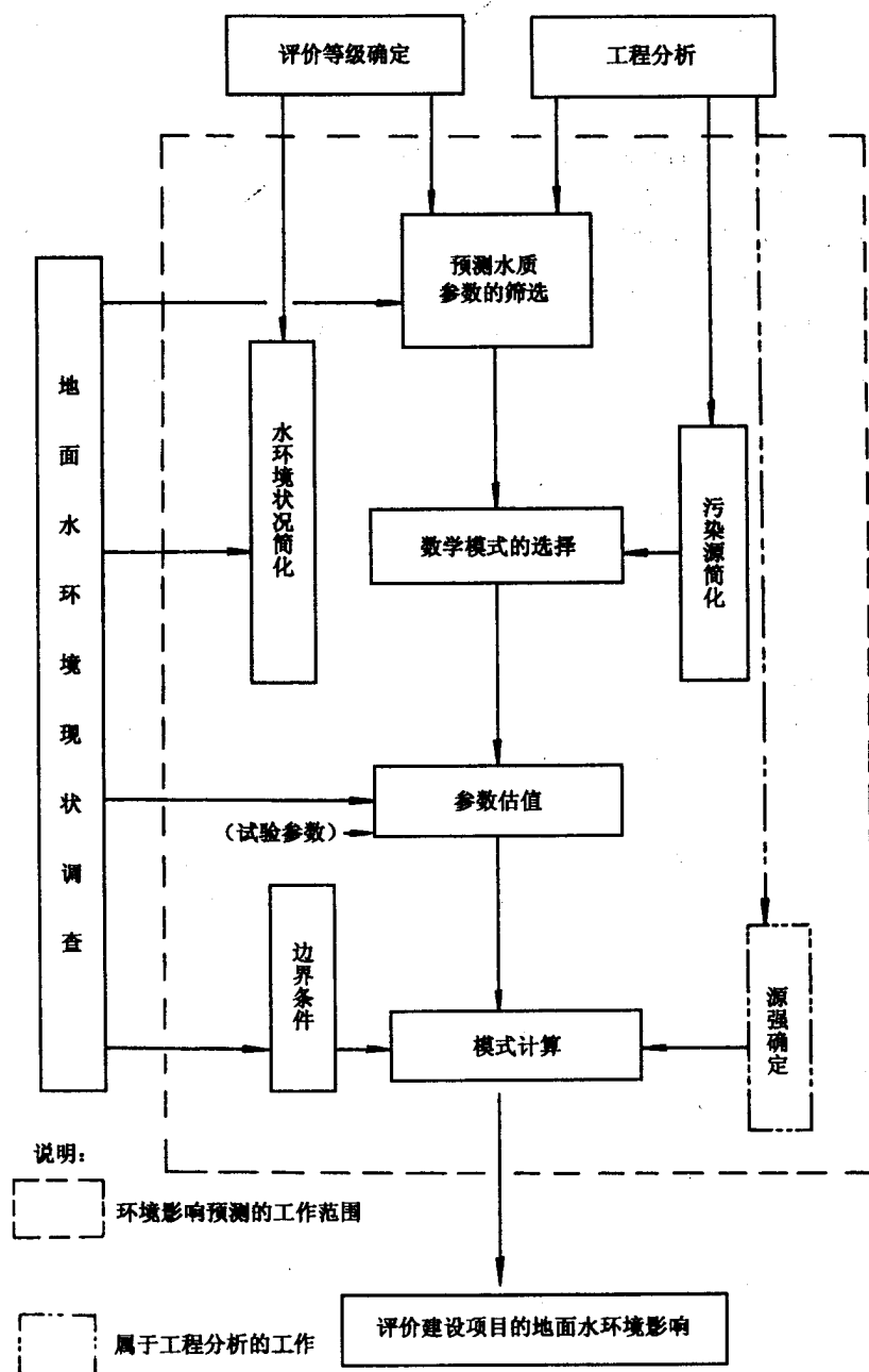
图2 采用数学模式法预测地面水环境影响的工作程序
