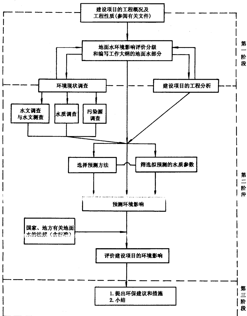
图1 地面水环境影响评价的工作程序
